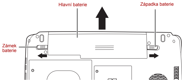
Uvolnění baterie
