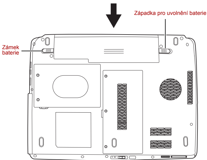
Zabezpečení baterie
