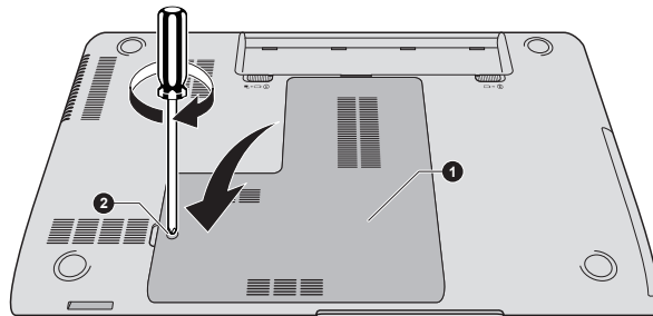
Obrázek 3-14 Usazení krytu paměťového modulu
