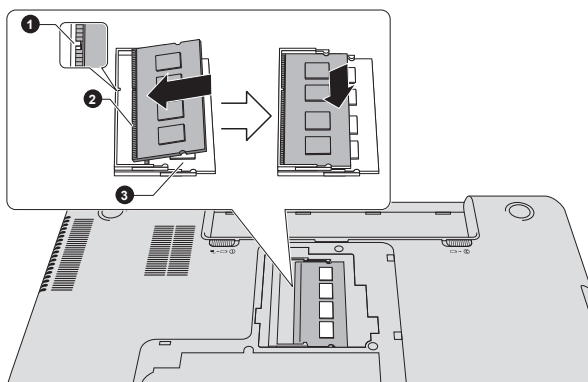
Obrázek 4-9 Usazení paměťového modulu
