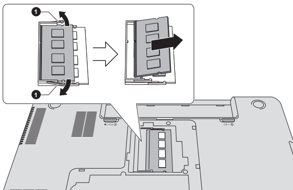
Obrázek 4-11 Vyjmutí paměťového modulu
