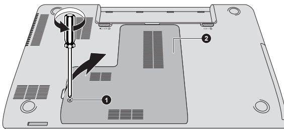
Obrázek 4-8 Sejmutí krytu paměťového modulu
