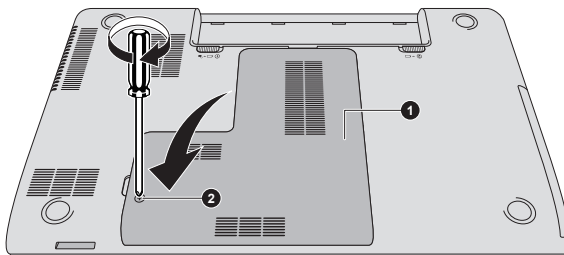
Obrázek 4-10 Usazení krytu paměťového modulu
