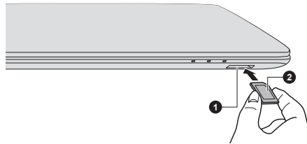
Obrázek 4-13 Vkládání paměťových médií
