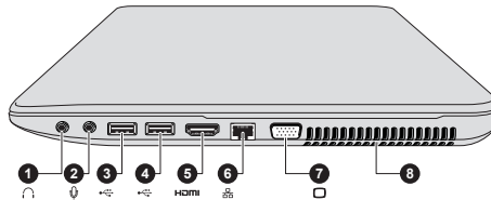
Obrázek 3-3 Pravá strana počítače
