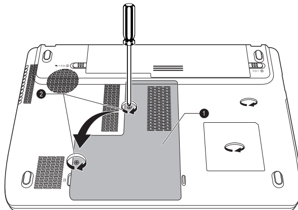
Obrázek 3-13 Usazení krytu paměťového modulu
