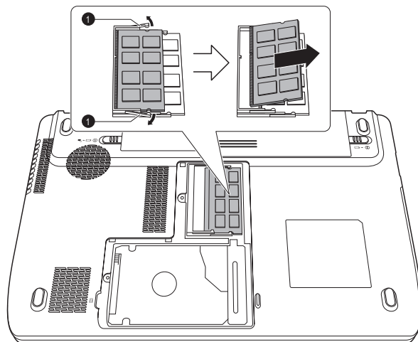
Obrázek 3-14 Vyjmutí paměťového modulu
