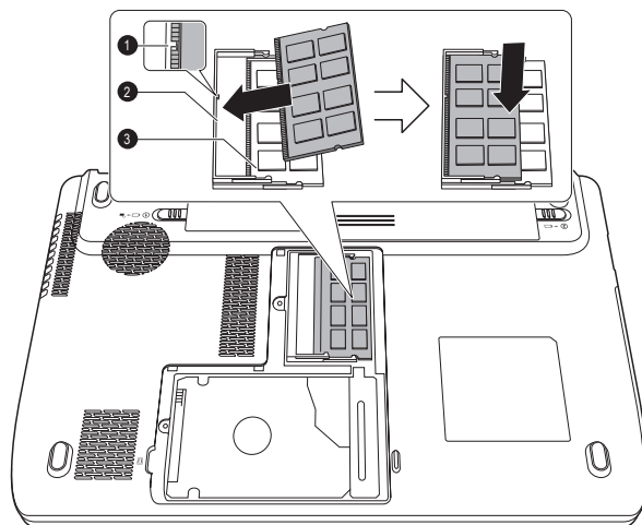
Obrázek 3-12 Usazení paměťového modulu
