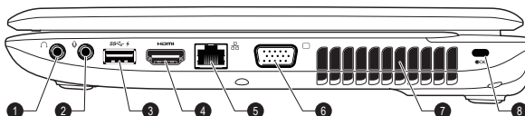
Obrázek 2-3 Pravá strana počítače
