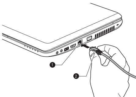
1. Konektor sítě LAN
