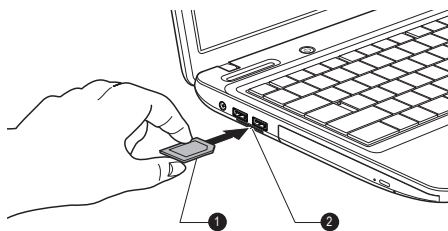
Obrázek 3-10 Vkládání paměťových médií
