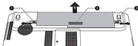
Obrázek 5-1 Uvolnění baterie
