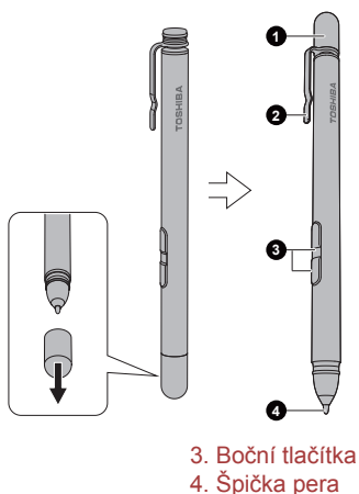
Obrázek 4-3 Stylus
