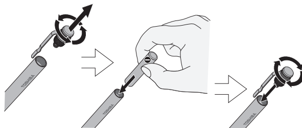
Obrázek 4-4 Instalace baterie
