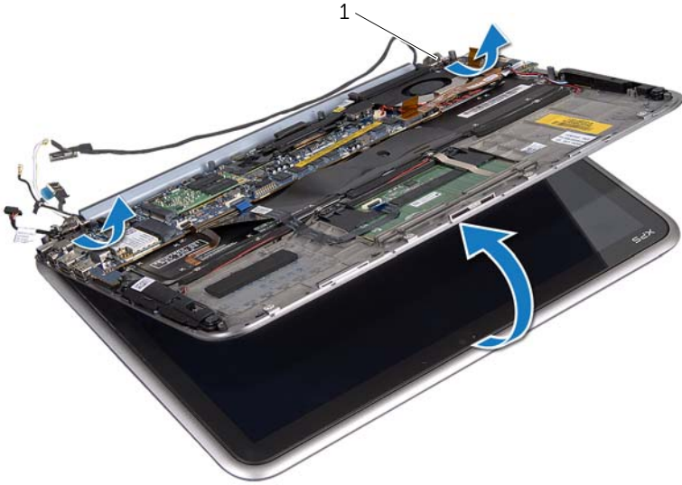
1 display hinges (2)
